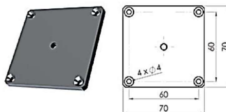
GROUND-PLATE 6063/SST
